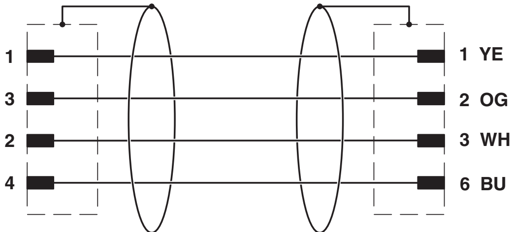
Schaltplan
