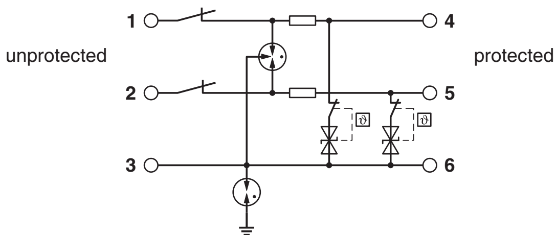
Diagrama eléctrico
