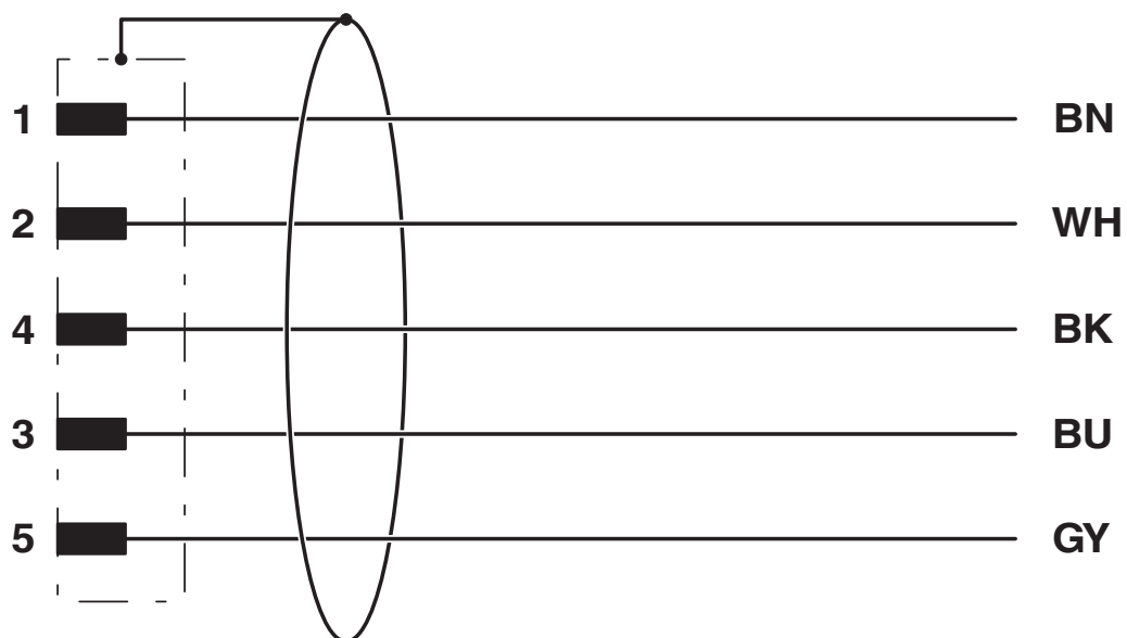
Kontaktbelegung der M12-Stecker
