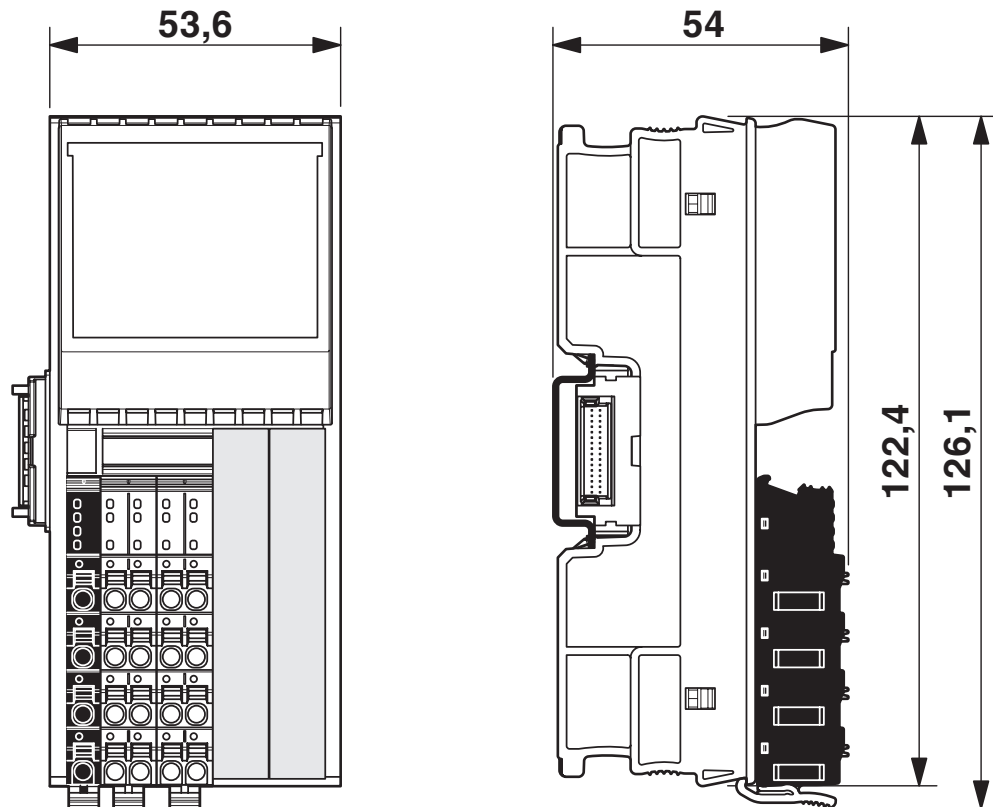
Dessin coté
