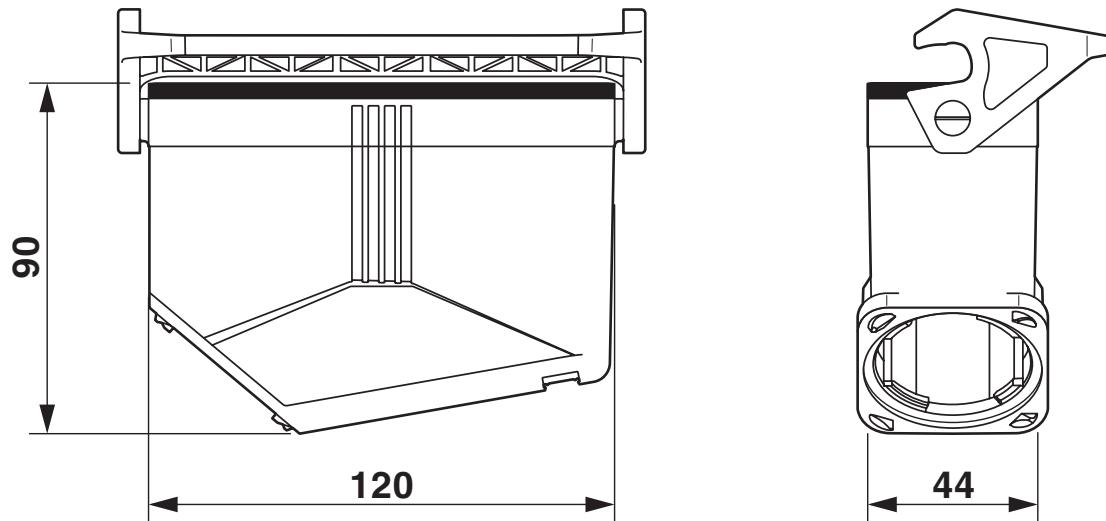
Maßzeichnung
