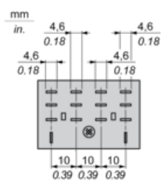
Stecker-Seitenansicht
