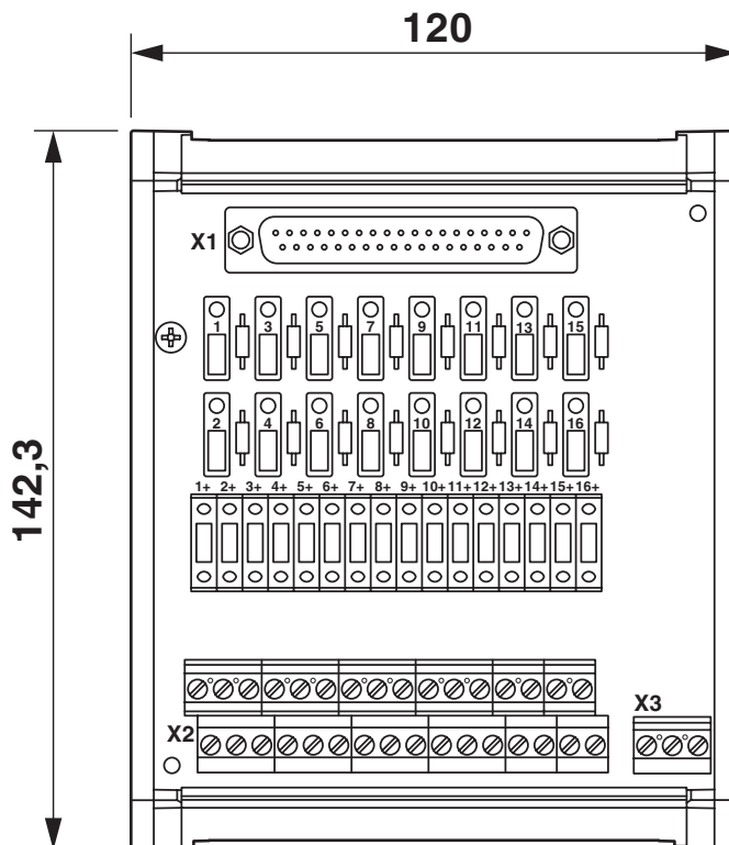
Maßzeichnung
