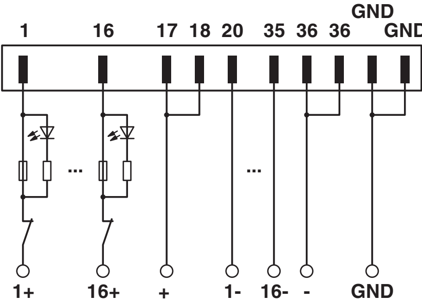
Diagrama eléctrico
