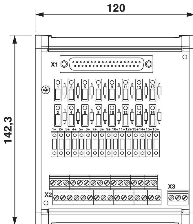
Dessin coté
