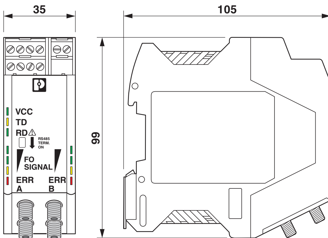
Dessin coté
