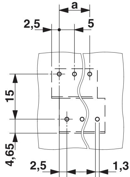
Bohrplan/Lötpadgeometrie
