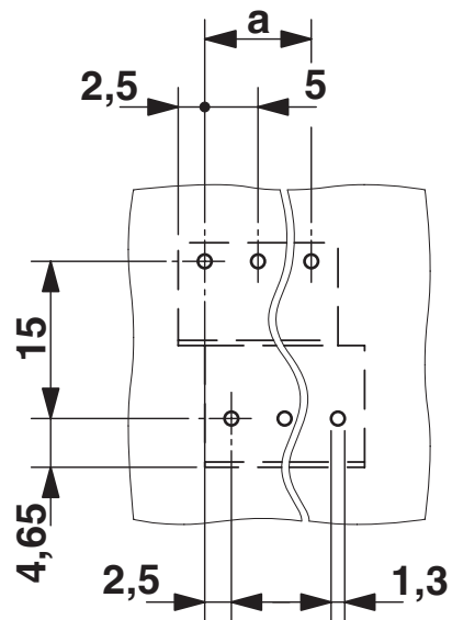
Esquema de taladros/geometría pads soldadura
