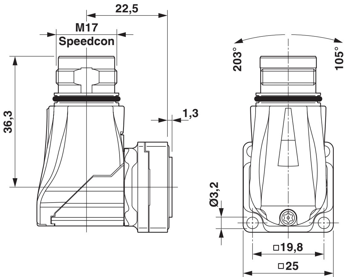
Maßzeichnung
