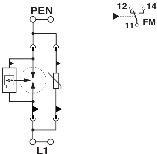
Diagrama eléctrico
