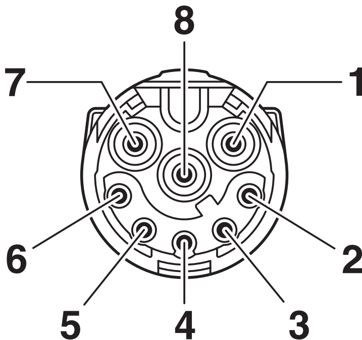
Plano esquemático
