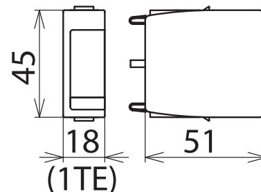
Maßbild DG MOD PV SCI 600
