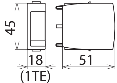
Maßbild DG MOD H NPE
