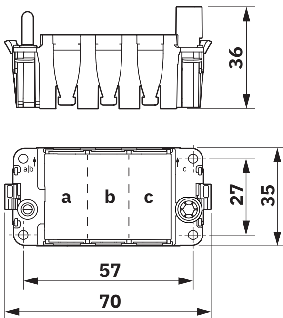
Maßzeichnung
