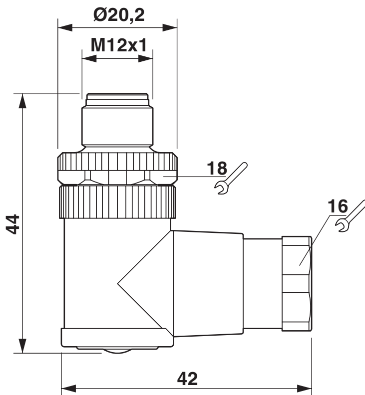
Dessin coté
