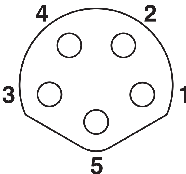
Esquema polos conector macho M8, 5 polos, codificado B, vista cara de machos
