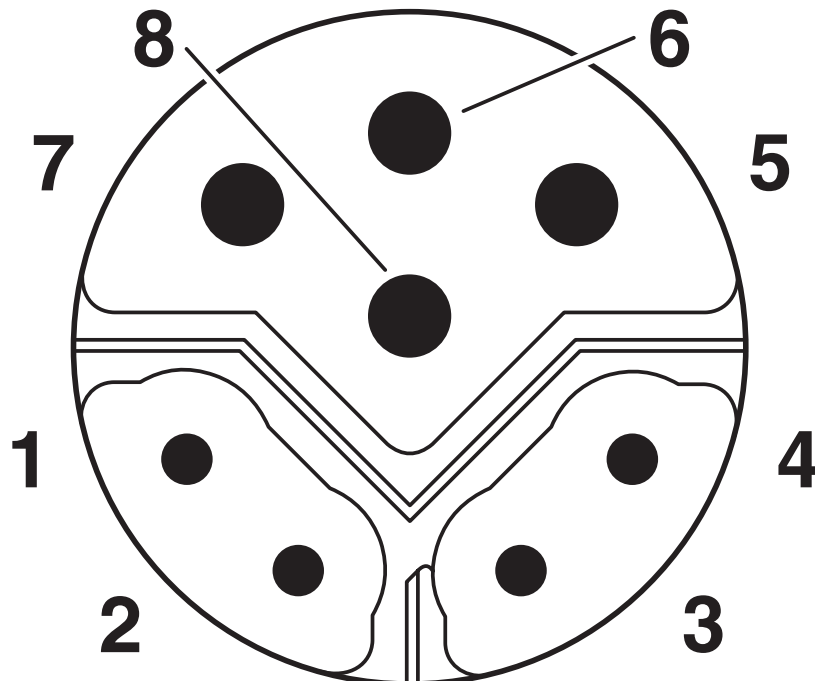
Schemazeichnung
