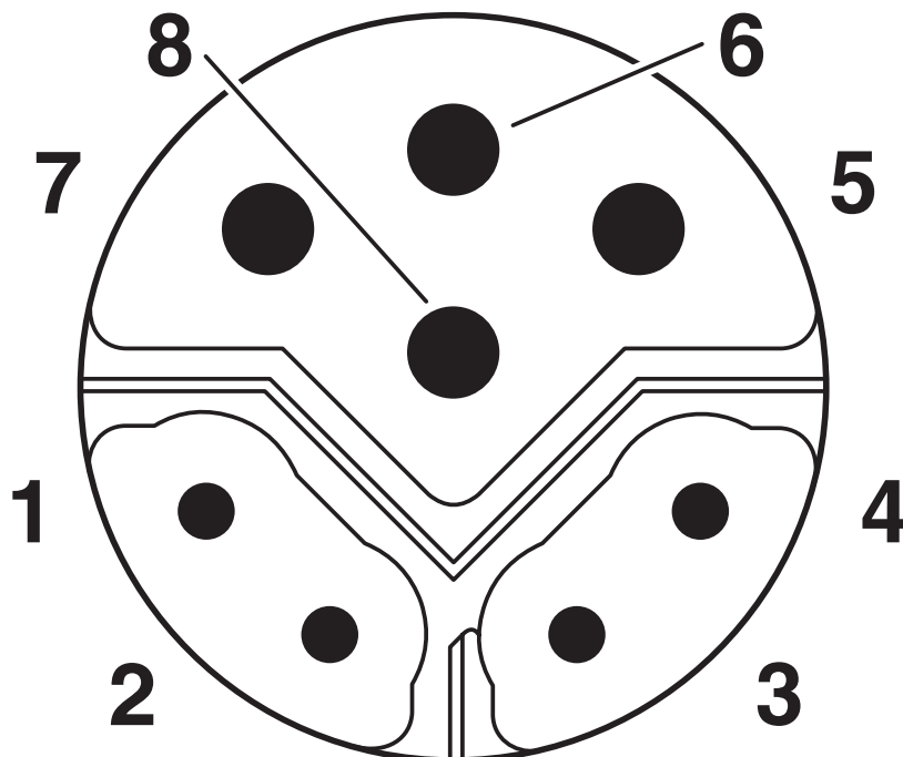
Esquema de polos conector híbrido M12 de 8 polos, codificado Y, vista lado macho
