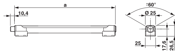
Maßzeichnung
