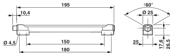
Maßzeichnung
