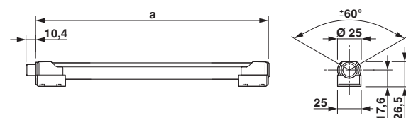
Dessin coté
