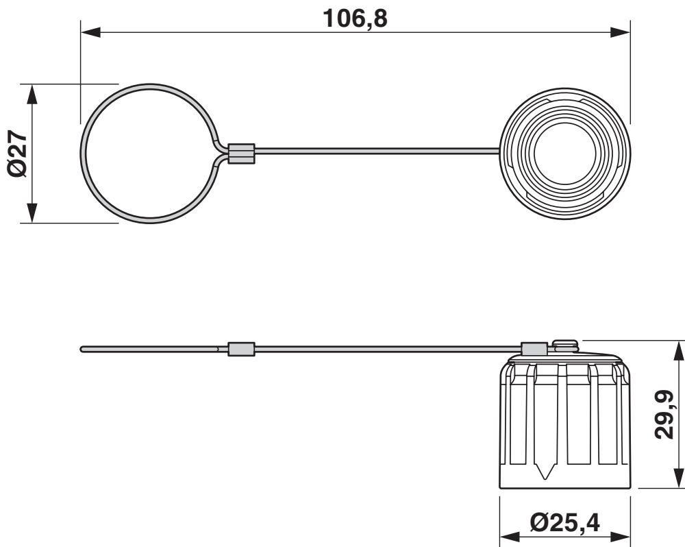
Maßzeichnung
