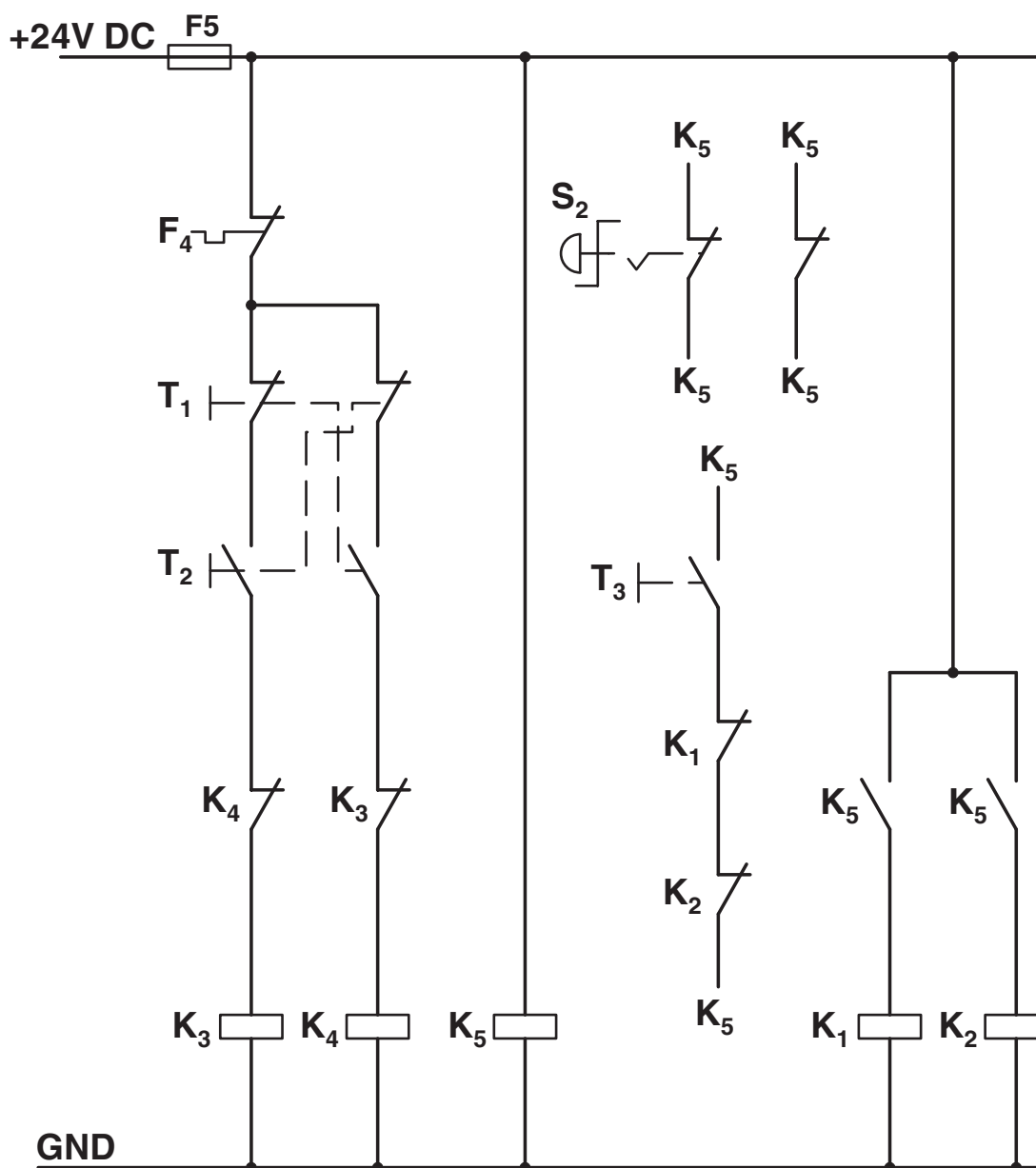
Schaltplan
