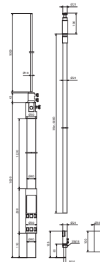
Maßbild HVI LI PL L6M SR1600 FSP1000 GFK
