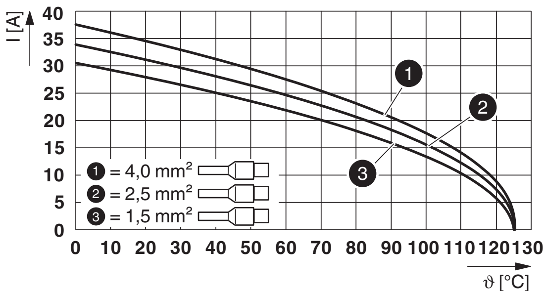
Diagramme de déclassement (à l'état non enfiché)
