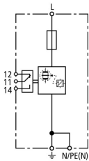
Esquema del DBM 1 CI 760 FM
