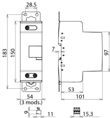
Dimensiones del DBM 1 CI 760 FM
