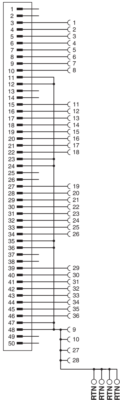
Schaltplan
