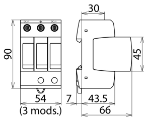
Dimensiones del DG M YPV SCI 1200
