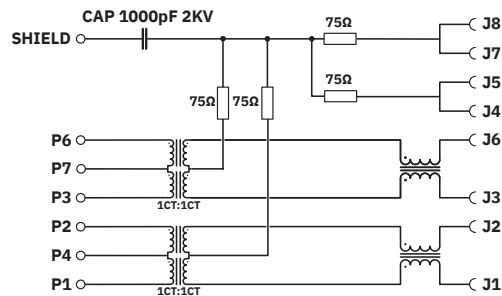
Schaltplan
