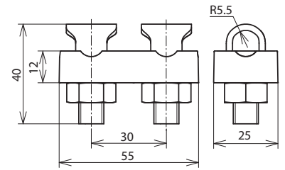
Maßbild KSV 2X7.10 STTZN
