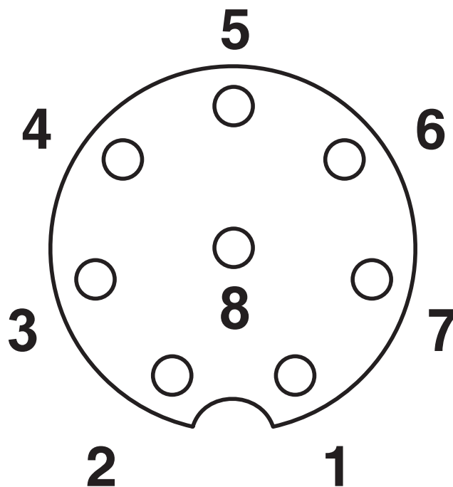
Esquema de polos del conector hembra M12, 8 polos, con codificación A, vista: lado del conector hembra
