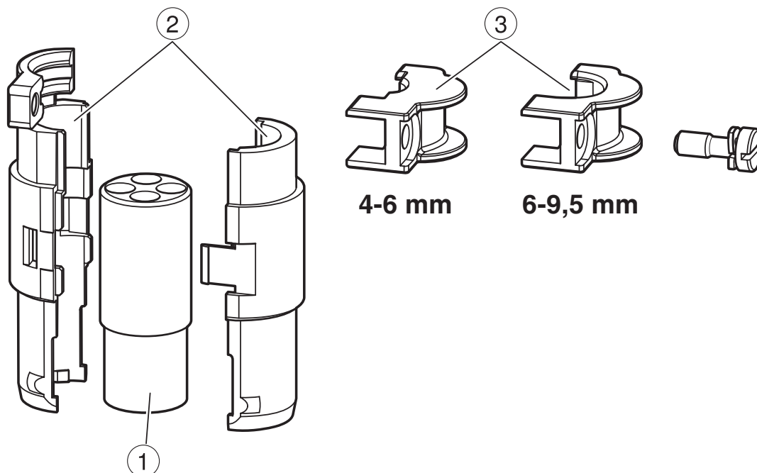
Dibujo funcional
