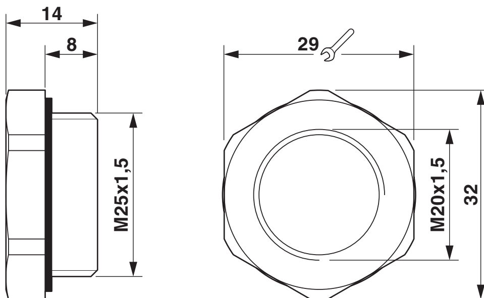
Dessin coté
