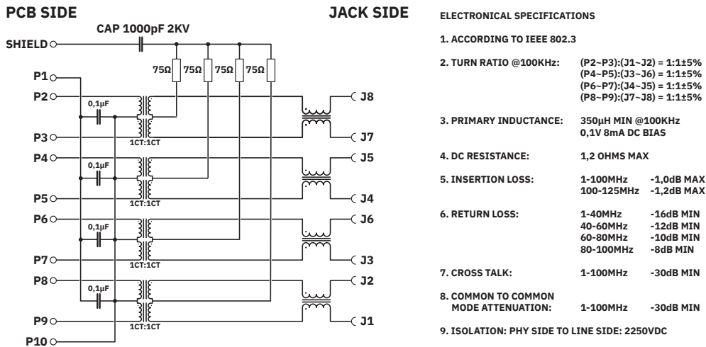
Diagrama eléctrico
