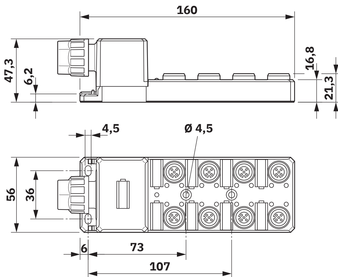
Dessin coté
