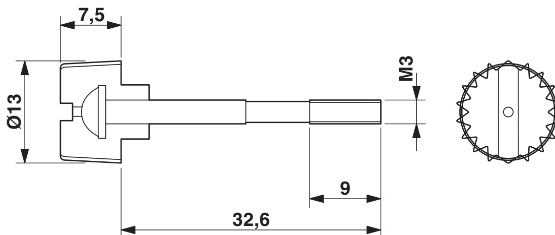
Dessin coté
