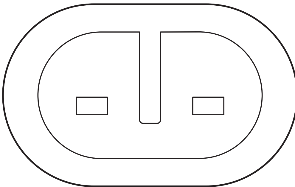
Esquema de polos, conector Super Seal, de 2 polos
