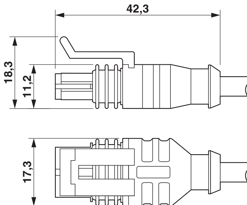
Superseal, conector hembra, vista superior y lateral
