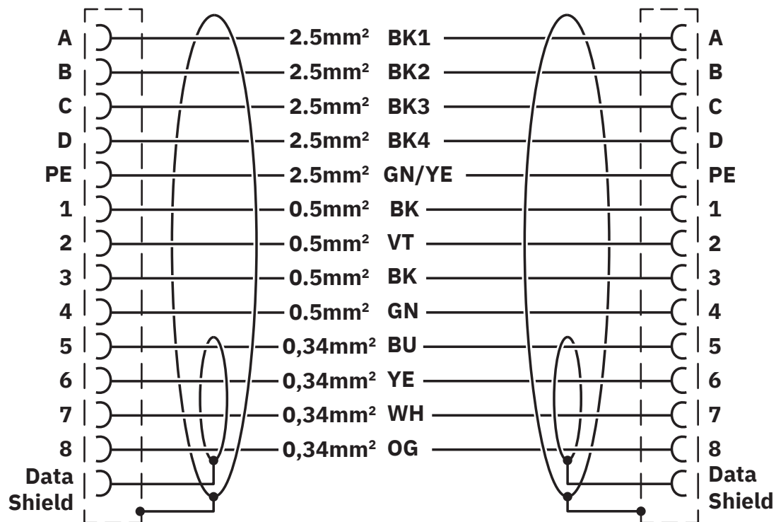
Diagrama eléctrico
