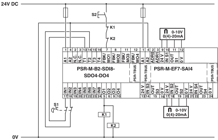
Applikationszeichnung
