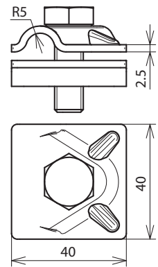
Maßbild MVK 8.10 M10 V2A
