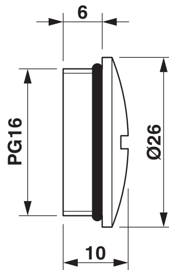
Maßzeichnung
