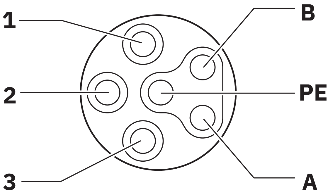
Schemazeichnung
