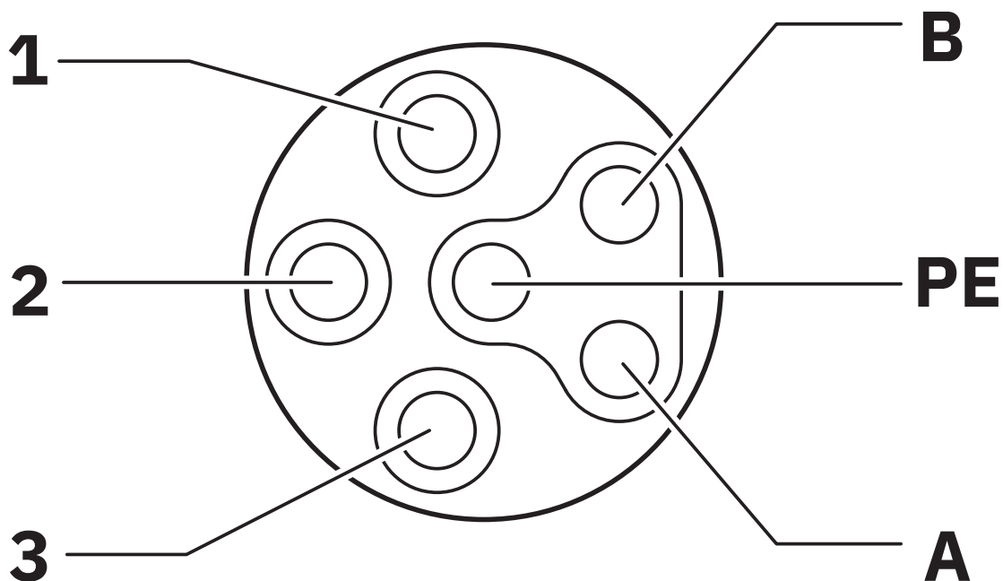
Esquema de polos de conector hembra S15 acodado a la derecha 270°, 6 polos, vista: lado de hembras
