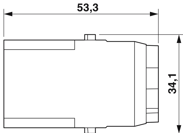
Maßzeichnung
