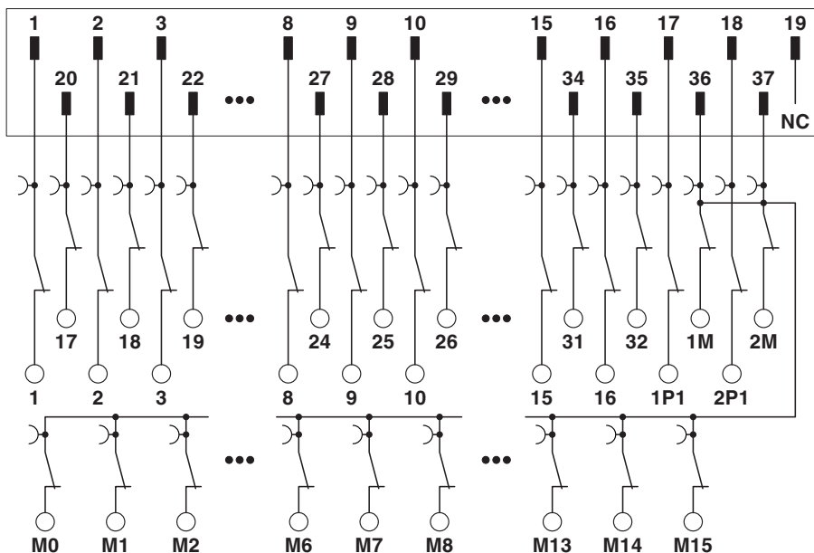
Schaltplan
