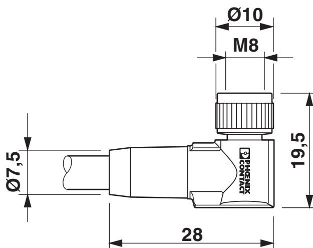
Dessin coté
