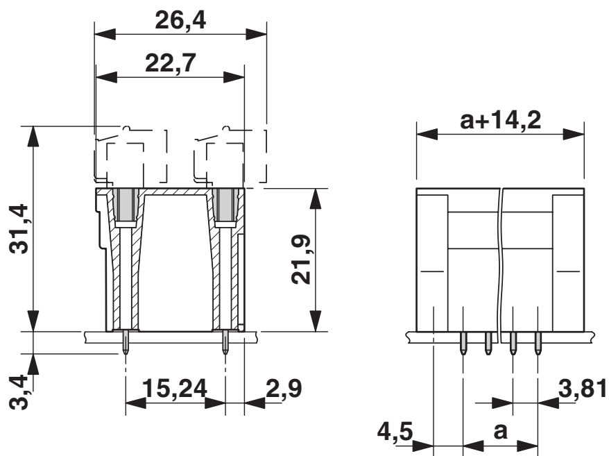
Dessin coté
